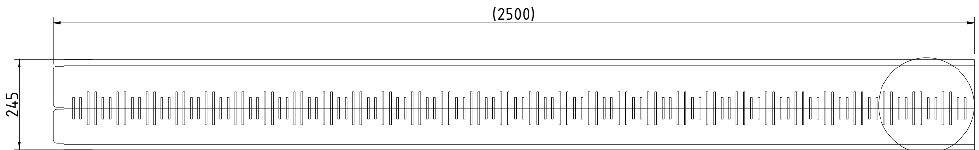
Abwicklung ( 1 : 10 )
